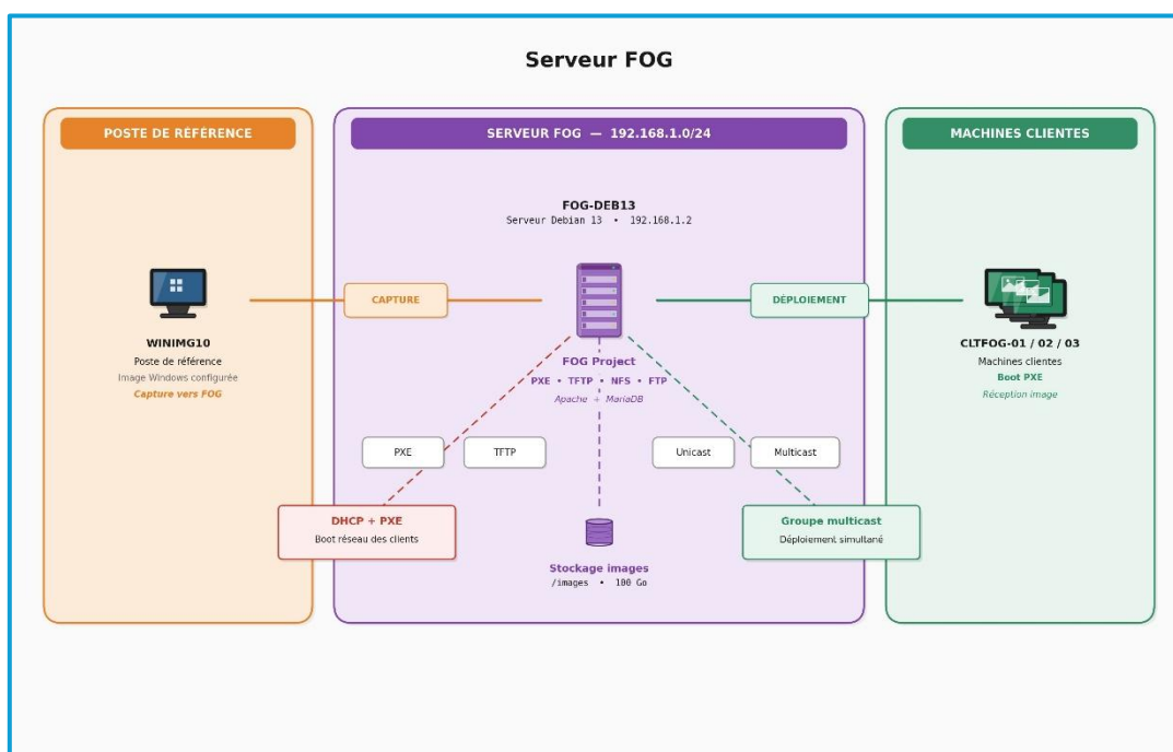
Schéma réseau :
